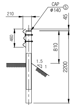
SIDE ELEVATION SCALE: NONE
