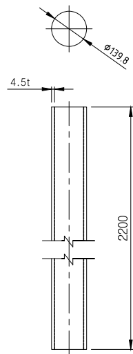
② Post SCALE: NONE
