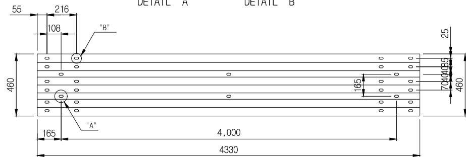
① 고규격가드레일 SCALE: NONE
