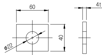
④ 사각와셔 SCALE: NONE
