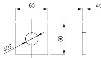
④ 사각와셔 SCALE: NONE
