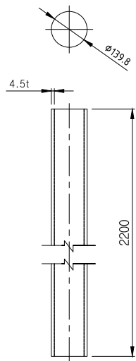
② 가드레일지주 SCALE: NONE
