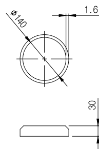
⑤ 주주캡 SCALE: NONE
