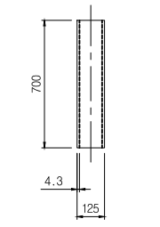
지주보강재 SCALE: NONE
