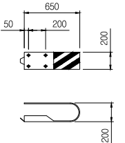
라운드레일 SCALE: NONE
