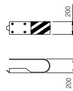
라운드레일 SCALE: NONE
