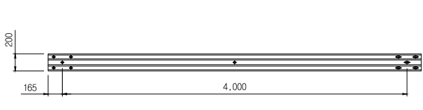
개방형 레일 SCALE: NONE
