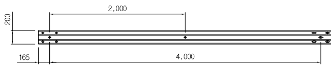
개방형 레일 SCALE: NONE
