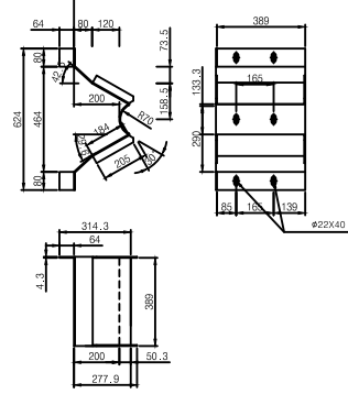
블럭아웃상세도
